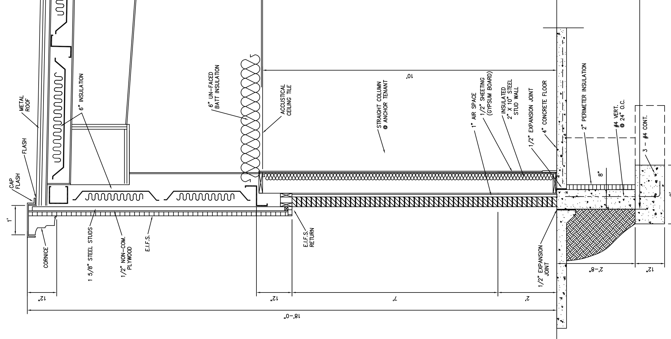
A DETAIL A SCALE: 1/2" = 1'-0"
