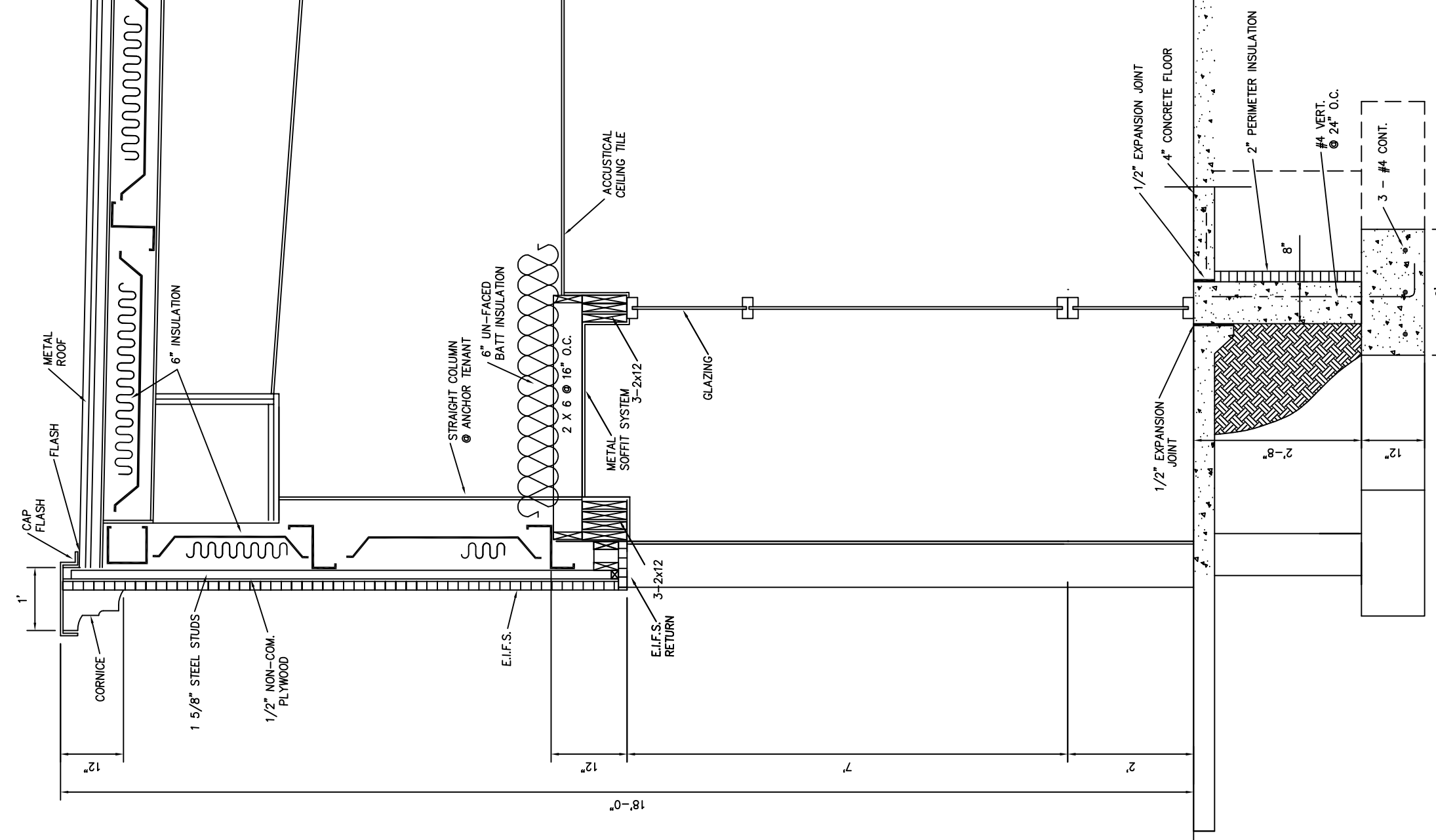
C DETAIL A SCALE: 1/2" = 1'-0"
