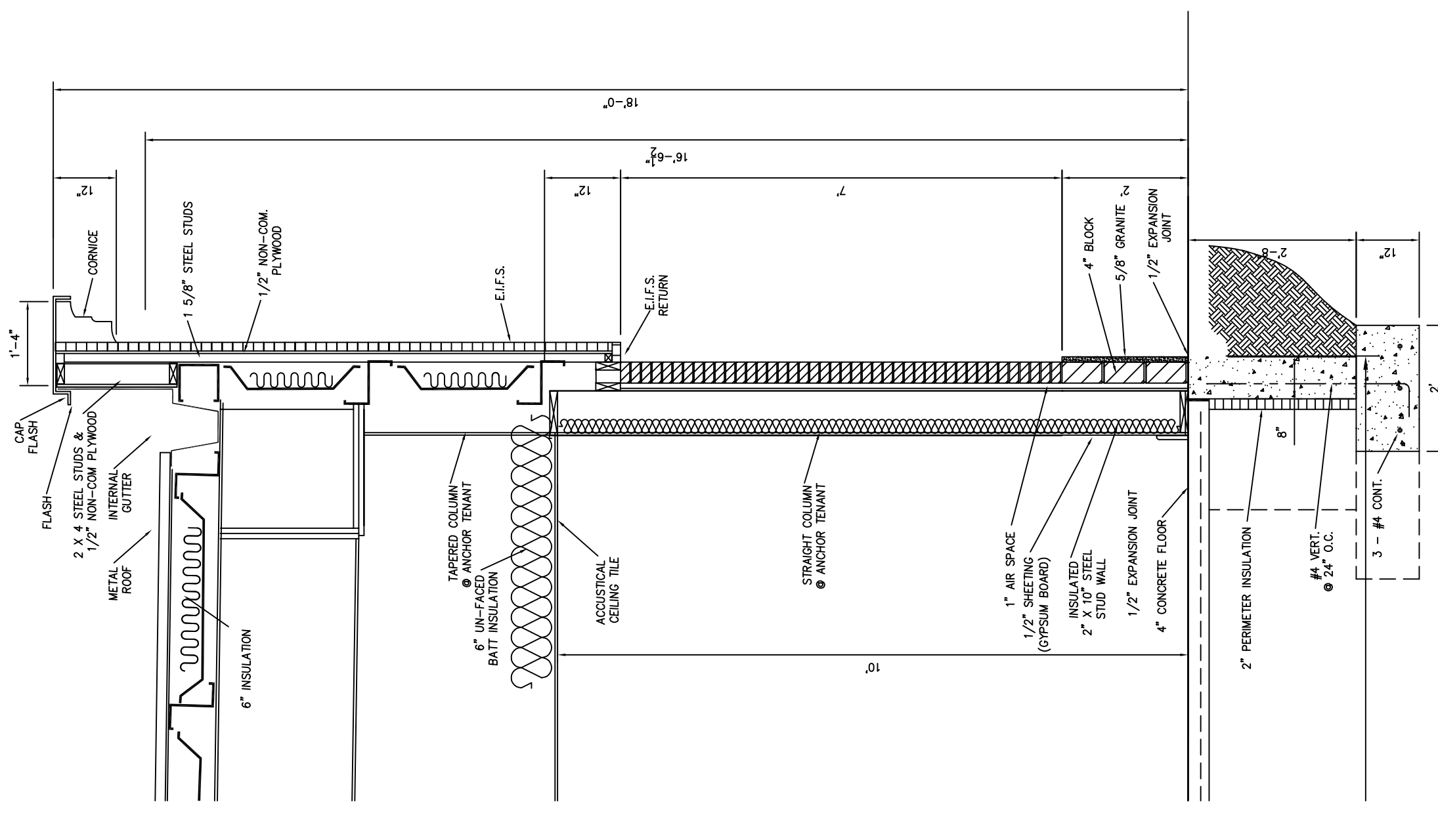
E DETAIL A SCALE: 1/2" = 1'-0"
